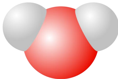
vattenmolekyl
